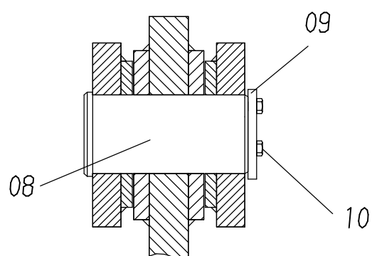
Schnitt B-B
