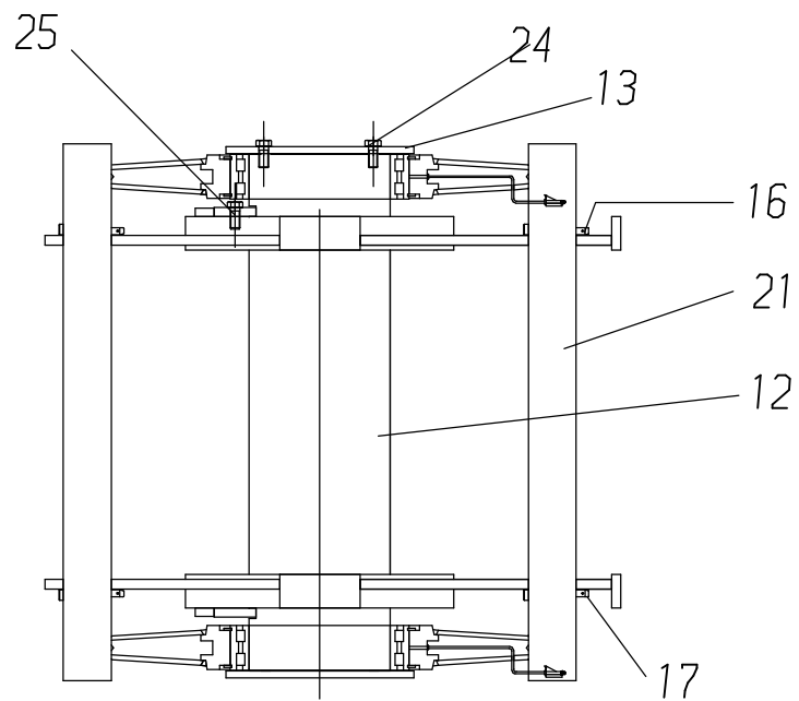
Schnitt A-A
