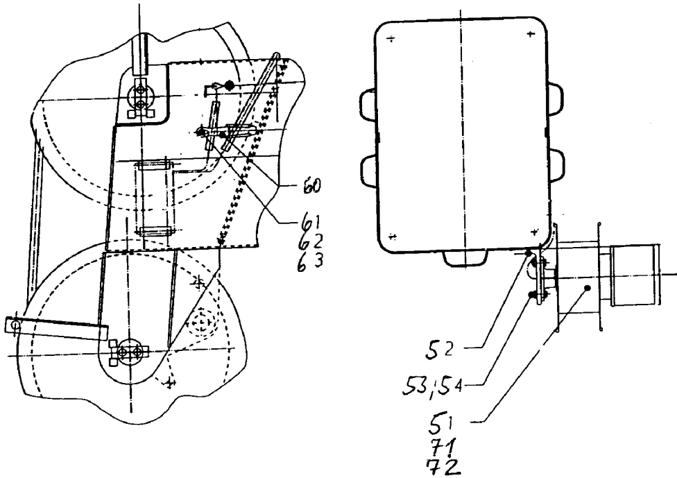
Schnitt B-B
