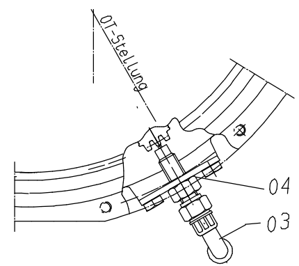
Anordnung des Drehzahlgebers am Kurbelwellengehäuse
