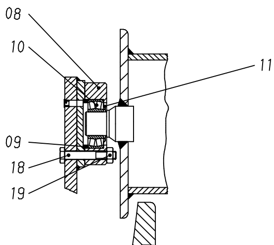
Schnitt C - C
