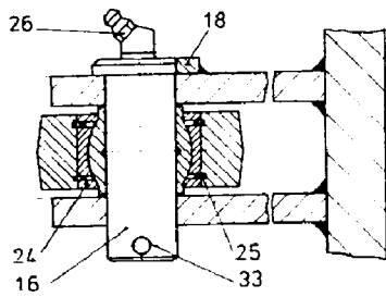
Schnitt C-C
