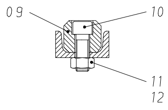
Schnitt C - D
