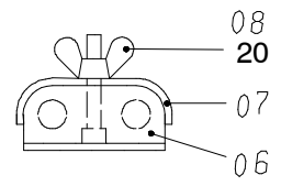
Einzelheit "X"
