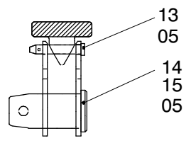
Schnitt G - H
