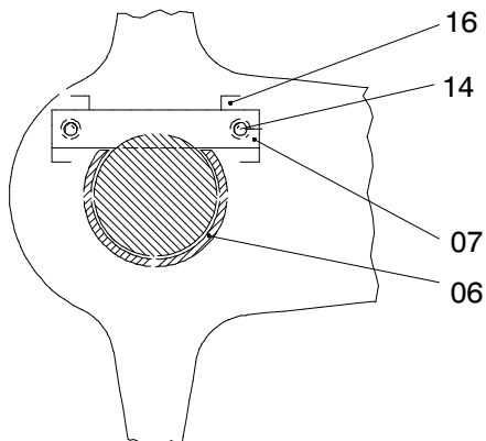
Schnitt A-A
