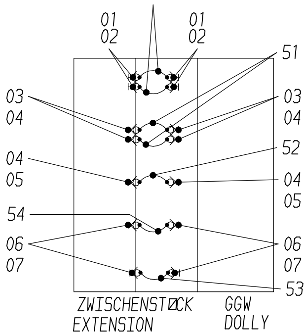
RAHMEN OBEN KURZ KPL TOP FRAME SHORT ASSY 50
