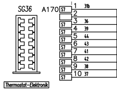
Thermostat-Elektronik
