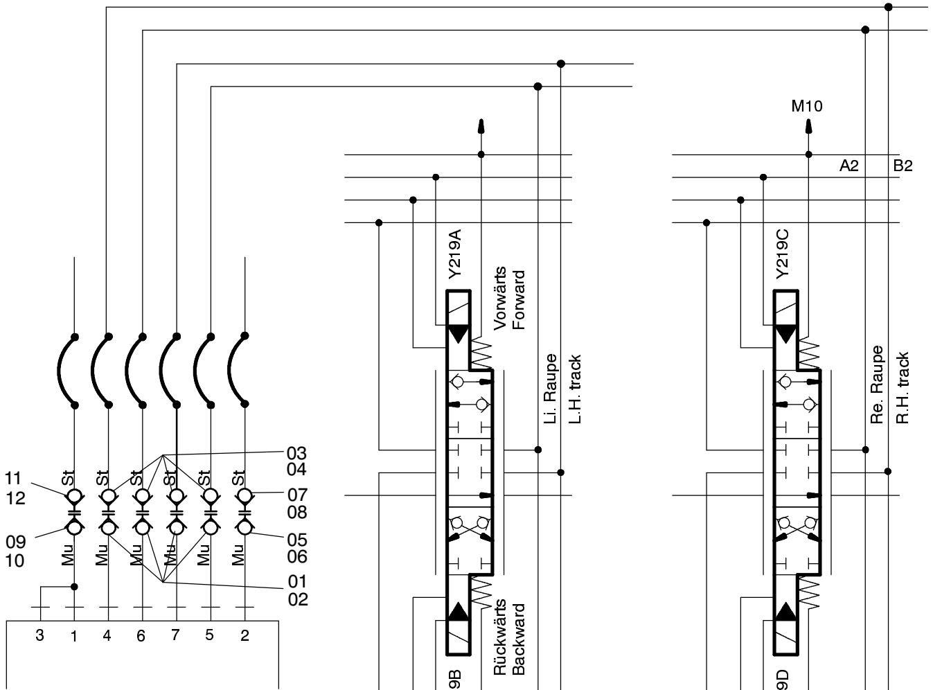
Drehdurchführung Rotary joint
