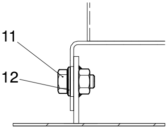
Einzelheit "Z"
