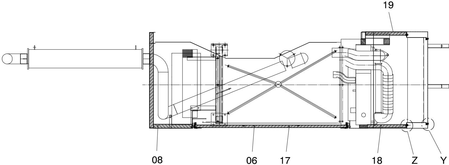
Ansicht X
