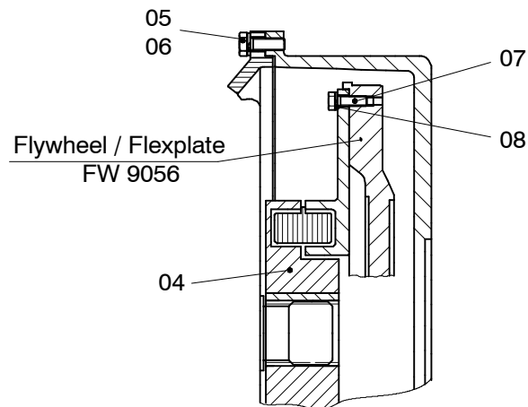
Schnitt A-A
