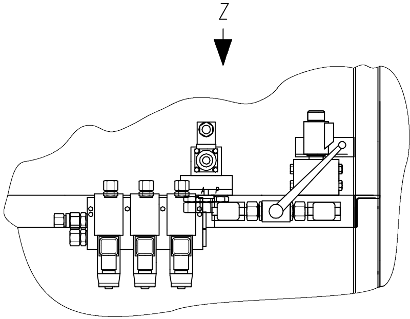
Ansicht Z
