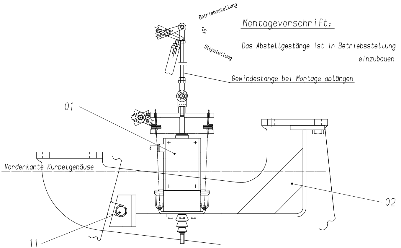
Motorstopmagnet und Halterung in Ansicht gezeichnet
