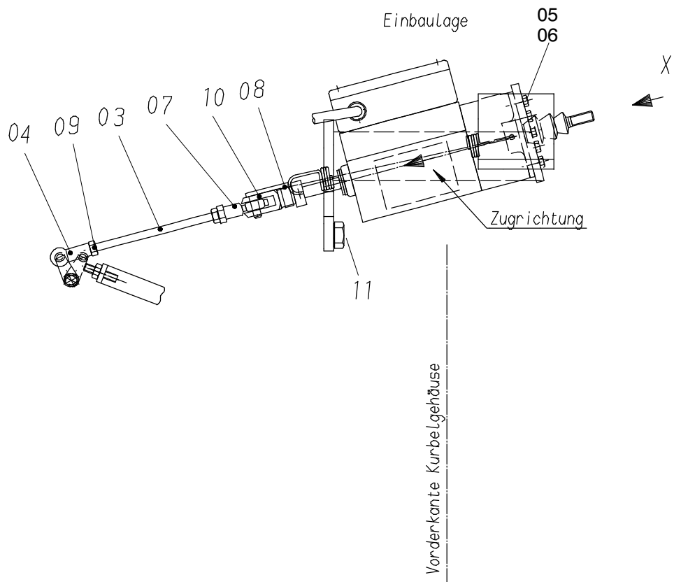
Motorstopmagnet und Halterung in Ansicht gezeichnet
