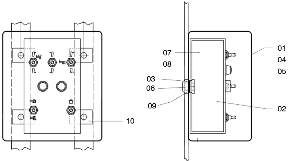
SCHNITT A-B
