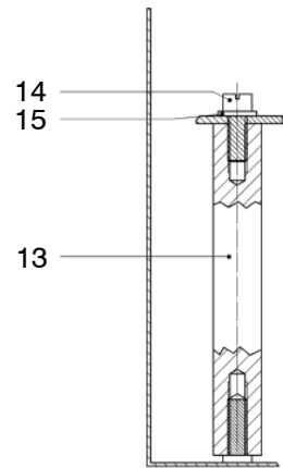
SCHNITT C-D
