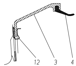
Schnitt B - B
