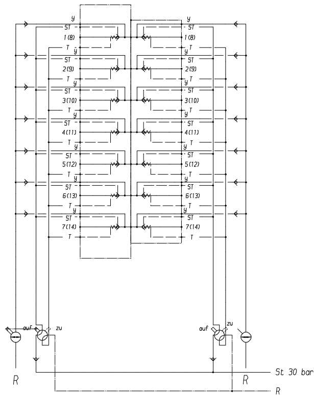
Schaltschema zeigt nur eine Ebene
