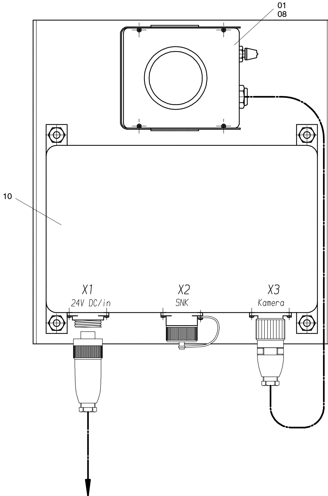
Verteilerkasten Hauptauslegerkopf Distributor Box, Main Boom Top
